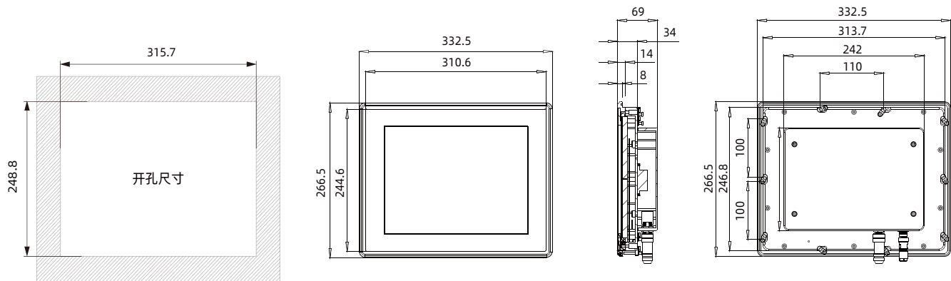
尺寸图 单位: mm
