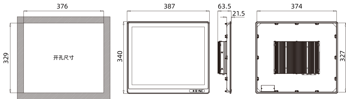
尺寸图 单位: mm
