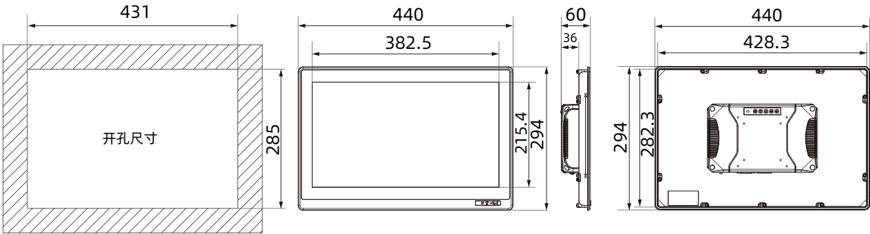
尺寸图 单位: mm
