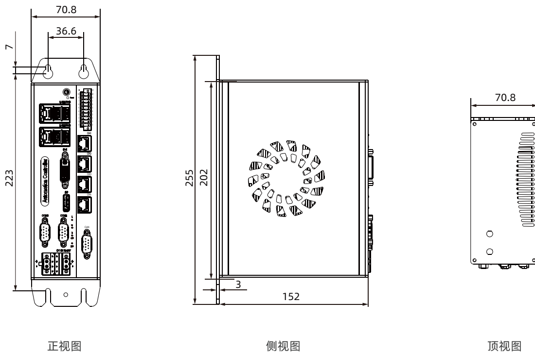
尺寸图 单位: mm
